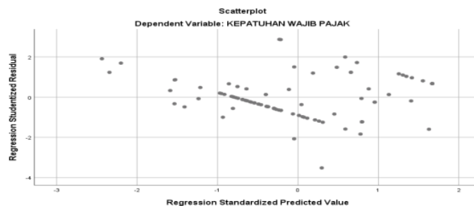
Gambar 1. Uji Heteroskedastisitas
