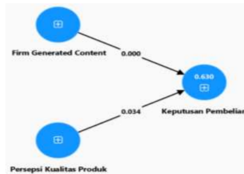
Gambar 1. Hasil Uji Boostrapping
